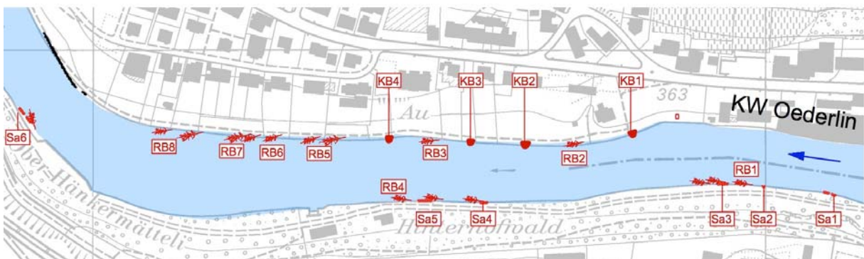
Bild 1: Standorte der Massnahmen, Massstab 1:4'000. RB: Raubaum, Sa: Ufersanierung, KB: Kleinbuhne.
